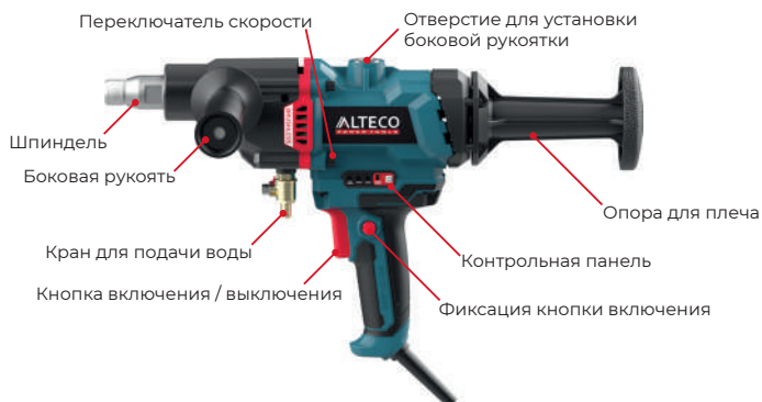
рис. 2. DD 26-200 GIK BL
